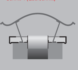
Schritt 4 (Querschnitt)
